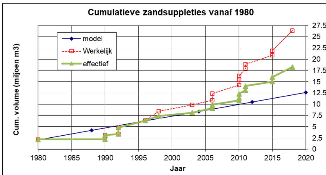
Figuur 3.1 Totale effectieve volume van de kustsuppleties op het Noordzeestrand van Ameland vanaf 1980
