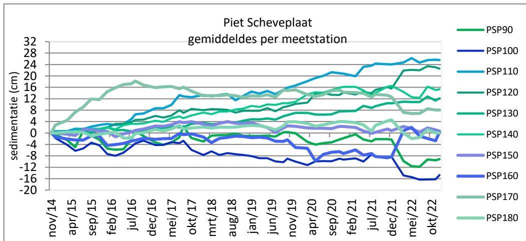
Figuur 6.27 Gemiddelde sedimentatie van de meetstations PSP90 t/m PSP180 in het onderzoeksgebied Piet Scheveplaat.
