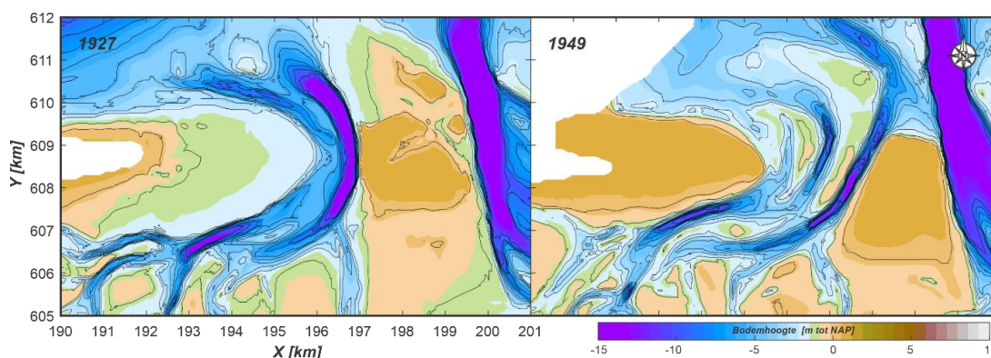
Figuur 4.2 Pinkegat in 1927 en 1949
