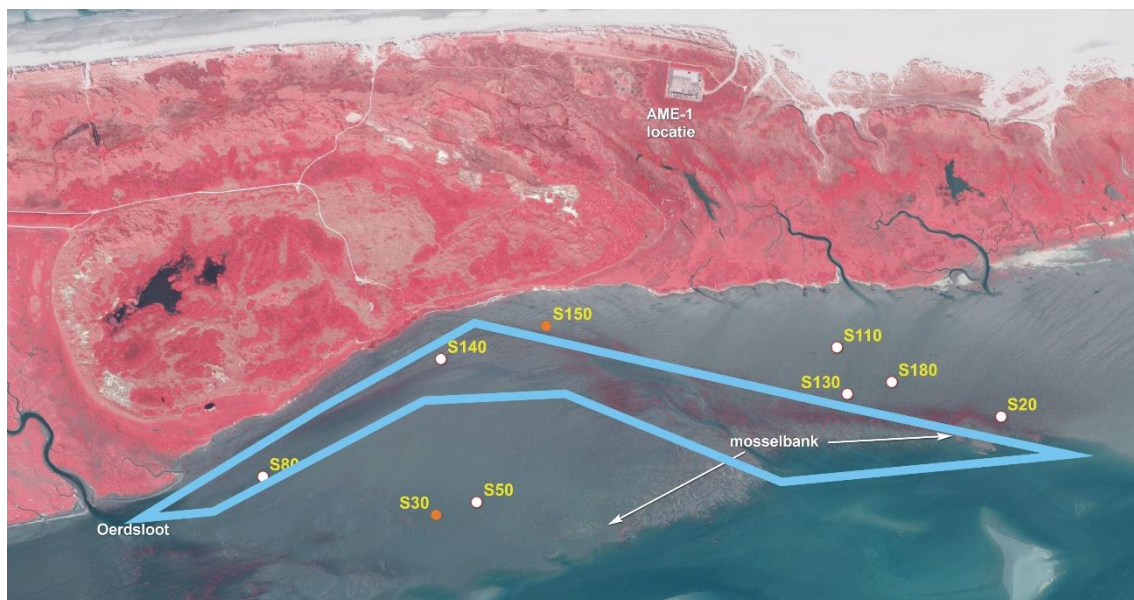
Figuur 6.18 De stations die met de witte stippen zijn gekleurd laten netto daling van het maaiveld zien ten gevolge van diepe daling door gaswinning. Het met blauw omlijnde gebied markeert globaal het gebied van netto maaiveld daling. Hierover stroomt/staat water tijdens lage waterstanden als de hogere delen zijn drooggevalen vanaf de monding van de Oerdsloot in oostelijke richting naar de eerste geul van het Pinkegat. Nieuw is een mosselbank die in 2021 op het zuidelijke deel van de wadplaat is ontstaan. Het gaat om ongeveer 20 ha over een lengte van ruim 1,5 km. De mossels waren in december 2022 ongeveer 3 tot maximaal 5 cm lang. Deze bank gaat mogelijk van invloed zijn op de afwatering en sedimentatie van het plaatgebied.
