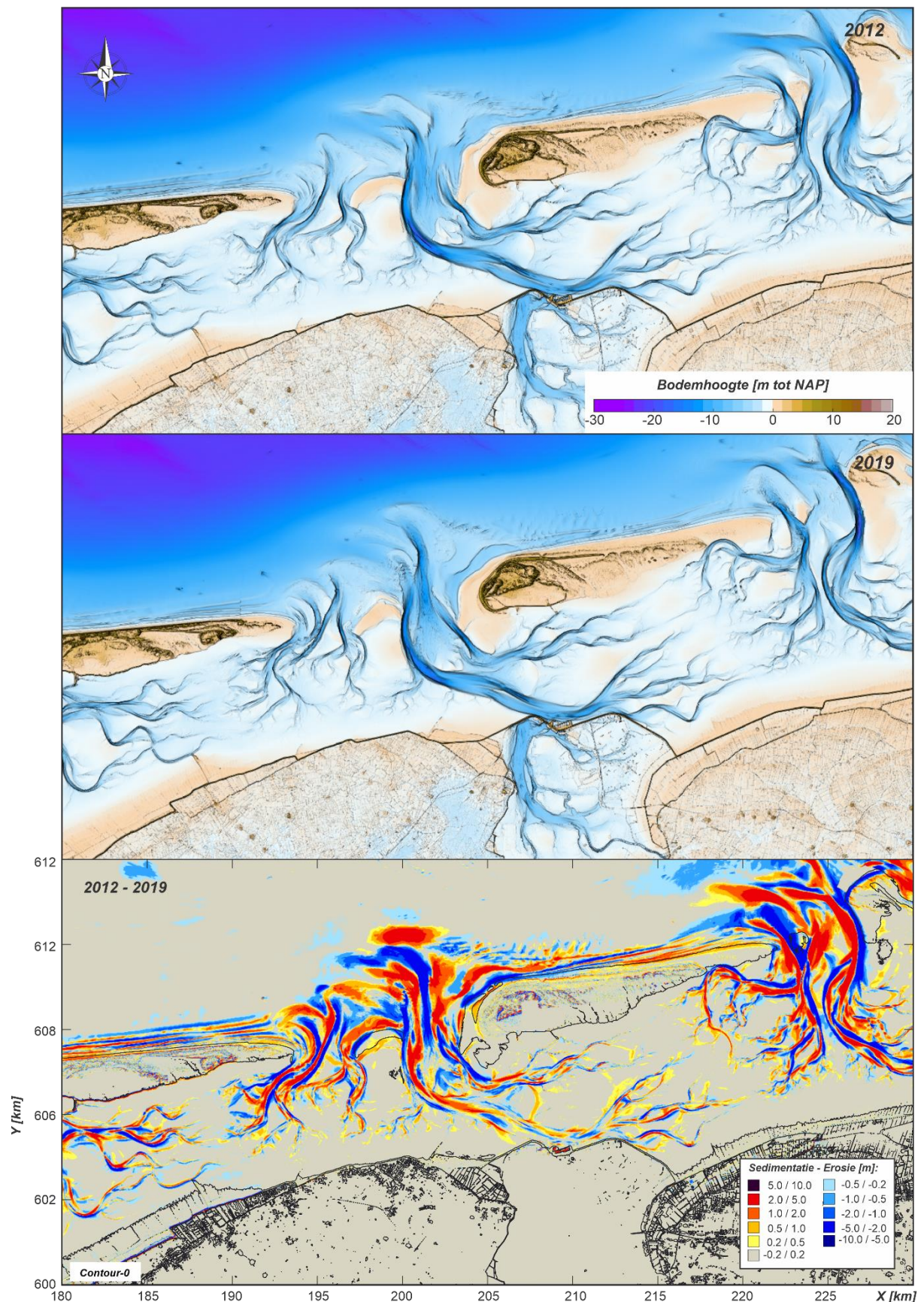
Figuur 2.6 Grootschalige morfologische ontwikkeling van het Friesche zeegat van 2012 tot 2019 op basis van de Vaklodingen. Het onderste plaatje toont de sedimentatie erosie patroon over deze periode.
