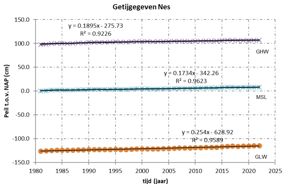
Figuur 10.3 Verloop moving-average (over de voorgaande 19 jaar) van gemiddeld hoogwater, gemiddeld zeeniveau en gemiddeld laagwater Nes
