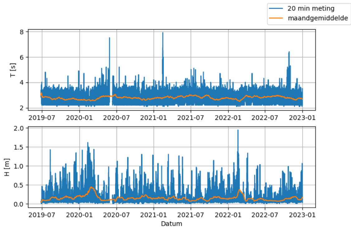
Figuur 10.7 Tijdseries van golfperiode (boven) en golfhoogte (onder).
