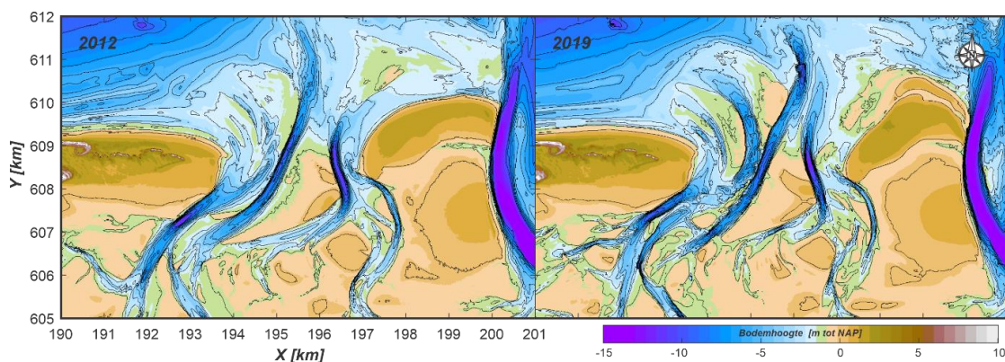
Figuur 4.7 Pinkegat in 2012 en 2019
