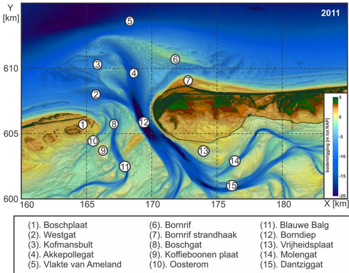
Figuur 2.3. Overzicht van de belangrijkste geulen en platen in het Amelanders zeegat
