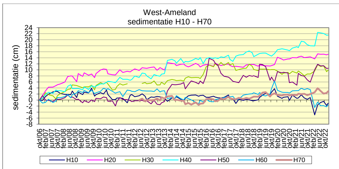
Figuur 6.22 Gemiddelde sedimentatie van de meetstations H10 t/m H70 in het onderzoeksgebied West-Ameland.
